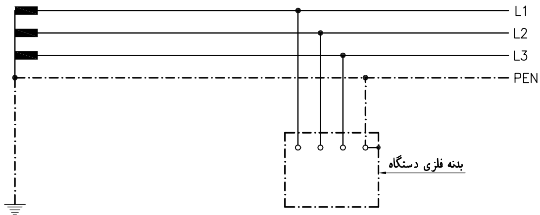
شکل شماره (۶-۱۲): سیستم اتصال زمین نوع TN-C کاربری بهینه: شبکه های محدود با بارهای عمدتاً سه فاز
