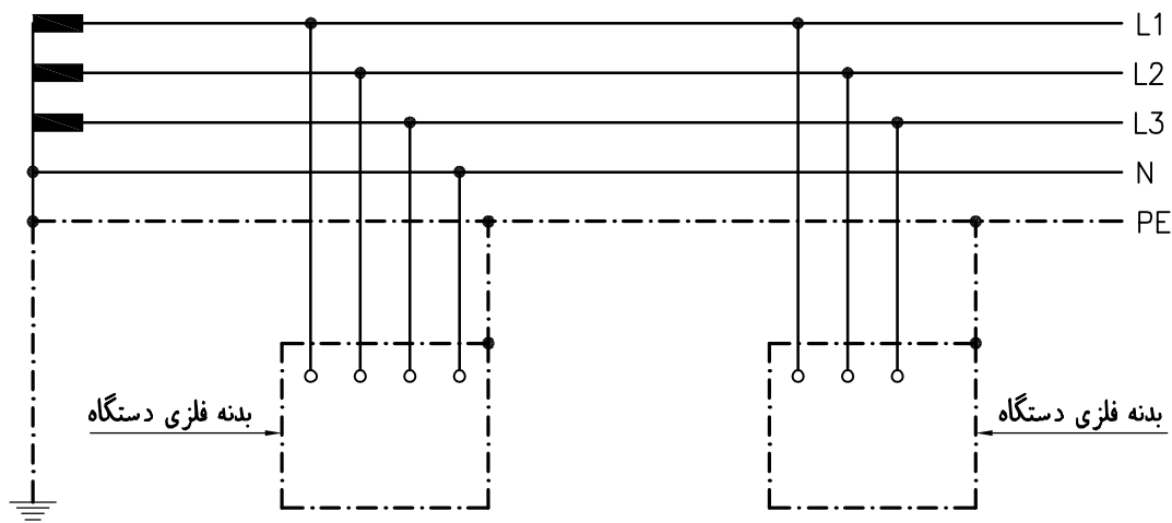
شکل شماره (۷-۱۲): سیستم اتصال زمین نوع TN-S کاربری بهینه: شبکه های محدود با بارهای تک فاز سه فاز
