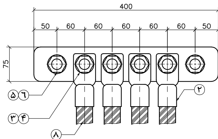
شین زمین از روی دیوار
