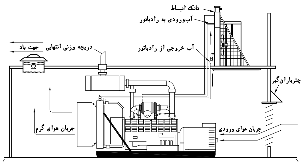
شکل شماره (۷-۷) - رادیاتور جدا از مولد
