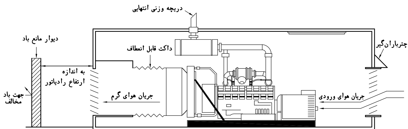
شکل شماره (۵-۷) - مسیر هوای خنک کننده
