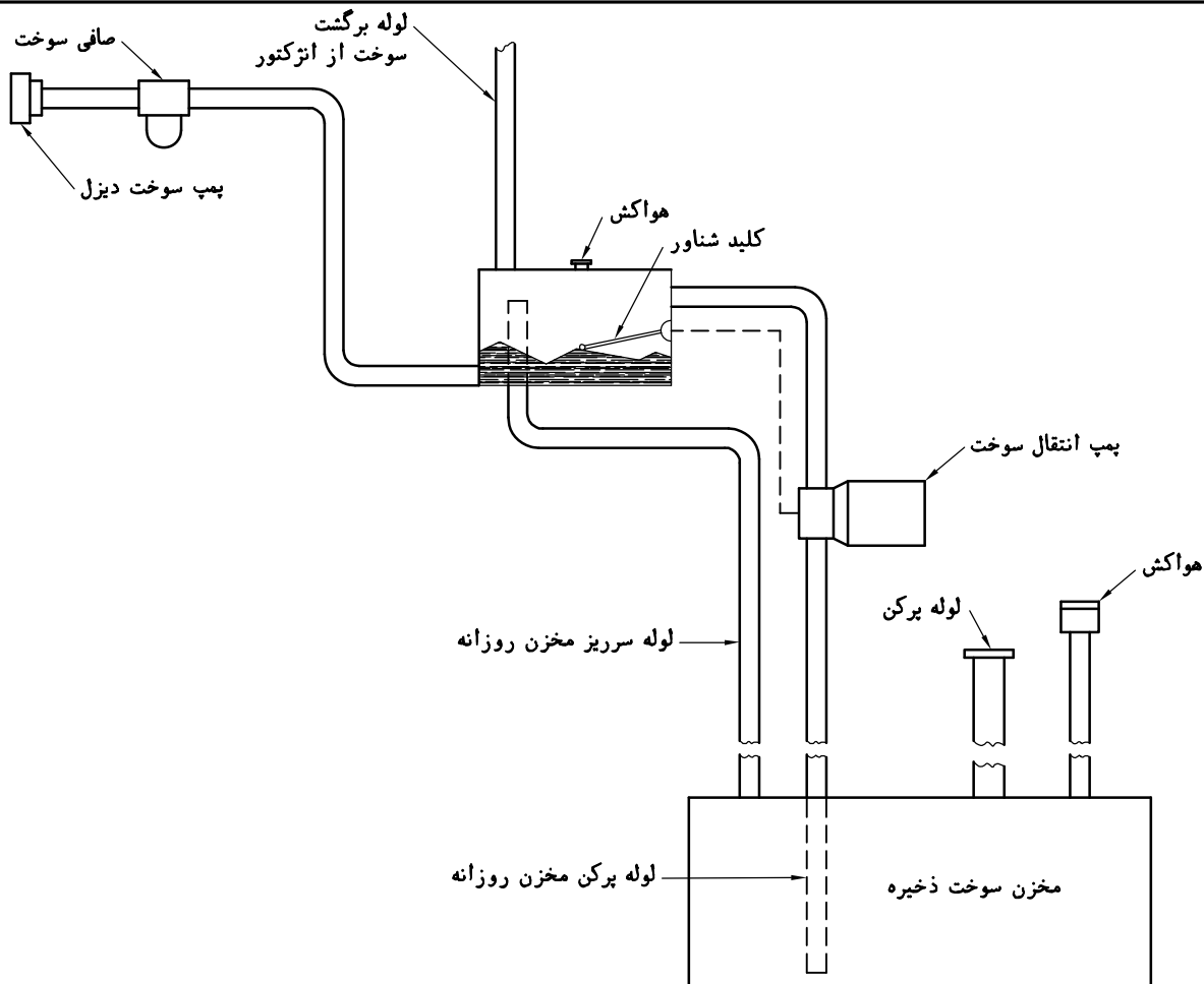
شکل شماره (۶-۷) - دیاگرام سوخت رسانی دیزل ژنراتور
