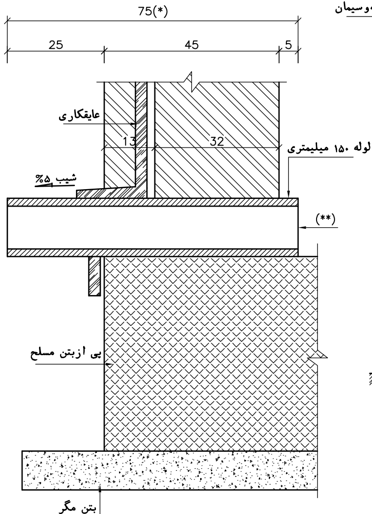
آرایش لوله و کابل فشار ضعیف در پست گکی (Sc: 1:10)
