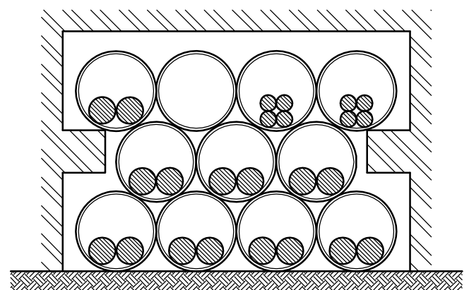
آرایش لوله و کابل فشار ضعیف در پست دوقاتی (Sc: 1:10)
