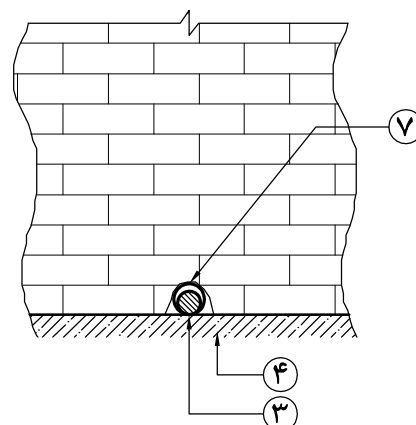
عبور لوله از زیر دیوار یا پارکینگ
